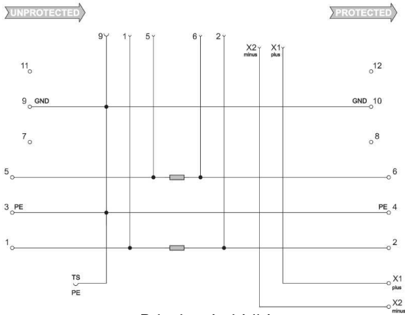
Prinzipschaltbild
