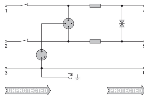
Prinzipschaltbild
