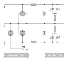
Prinzipschaltbild
