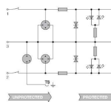
Prinzipschaltbild
