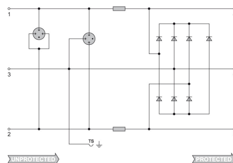
Prinzipschaltbild
