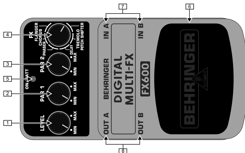
Oberseitenansicht
