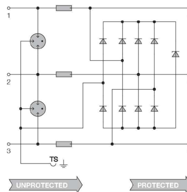
Prinzipschaltbild
