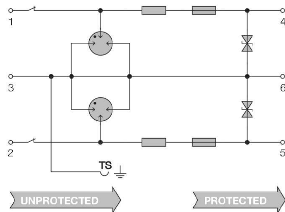
Prinzipschaltbild
