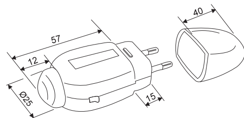
Bild 4: Abmessungen LED 2000, Typ 4052...
