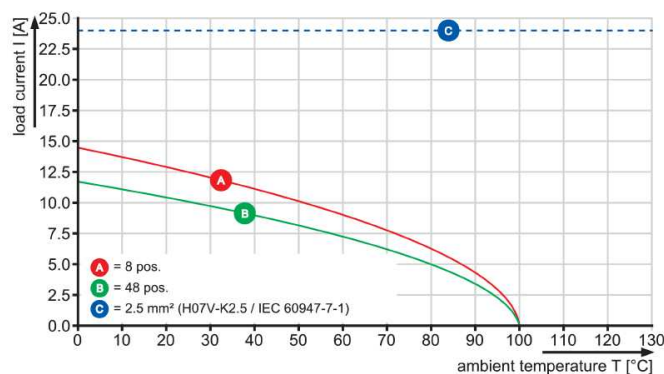
BLZP 5.08/./180 - SLDV-THR 5.08/./180
