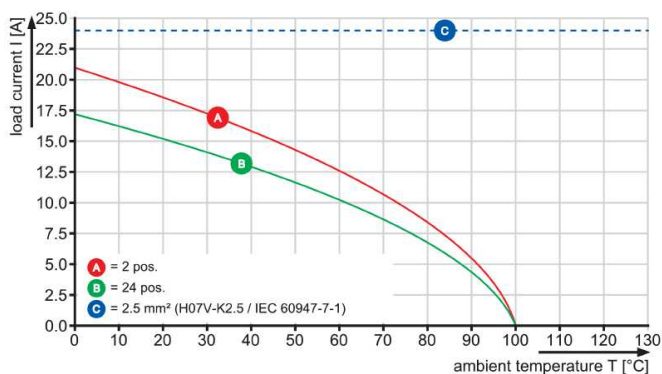
BLZP 5.08/./180 - SL 5.08/./90
