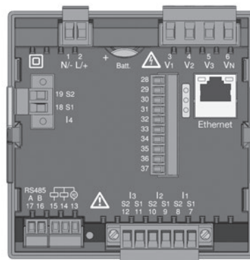
Rückansicht
