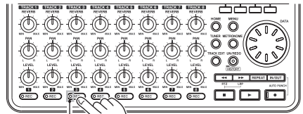
REC-Lämpchen von Spur 3
