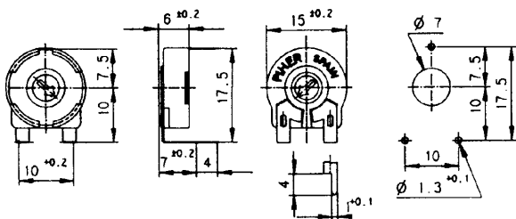
PT 15 Lv (17,5) PTC 15 Lv (17,5)
