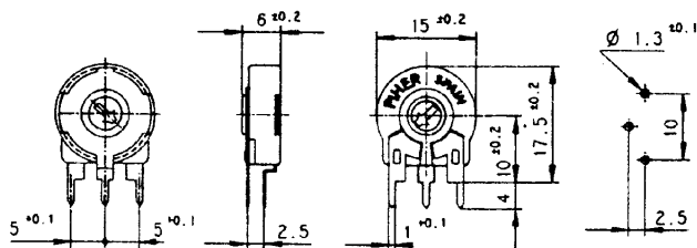
PT 15 Lh (2,5) PTC 15 Lh (2,5)
