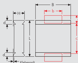
Lötpadempfehlung.
