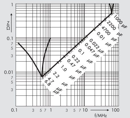
Scheinwiderstand in Abhängigkeit von der Frequenz (Richtwerte).
