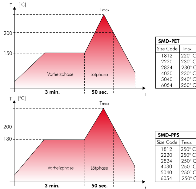
Temperatur/Zeitdiagramm für die zulässige Verarbeitungstemperatur der WIMA SMD-Reihen in einem typischen Konvektions-Lötverfahren.
