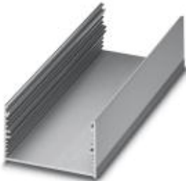
Aufbaugehäuse, Oberteil, Farbe: aluminium, Breite: 200 mm, Bauhöhe: 43,1 mm
