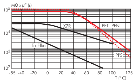
Isolationwert in Abhängigkeit von der Temperatur (Richtwerte)
