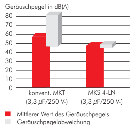
Streuung der Schallpegel-Messwerte
