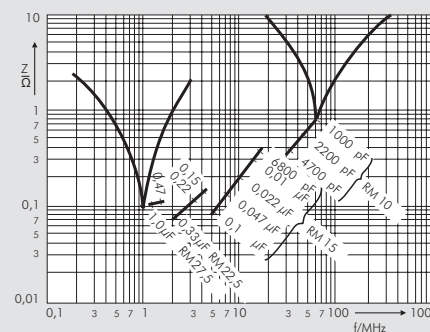
Scheinwiderstand in Abhängigkeit von der Frequenz (Richtwerte)
