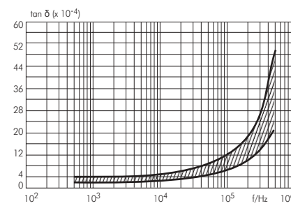
Verlustfaktor in Abhängigkeit von der Frequenz (Richtwerte).
