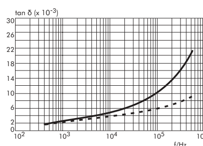
Verlustfaktor in Abhängigkeit von der Frequenz (Richtwerte)
