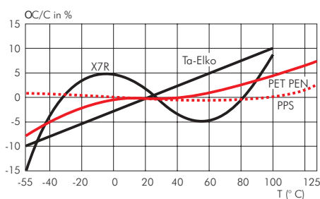
Kapazitätsänderung in Abhängigkeit von der Temperatur (f = 1 kHz) (Richtwerte)
