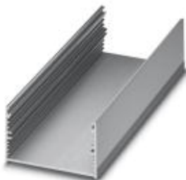
Aufbaugehäuse, Oberteil, Farbe: aluminium, Breite: 235 mm, Bauhöhe: 43,1 mm
