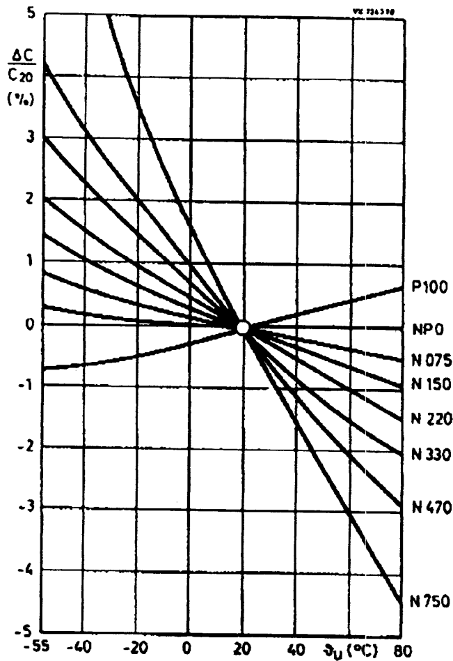
Bild 1 Kapazitätsänderung in Abhängigkeit von der Temperatur für Klasse 1-Kondensatoren mit Temperaturkoeffizienten von +100 \cdot 10^{-6} / \text{K} bis -750 \cdot 10^{-6} / \text{K} (P 100 bis N 750)
