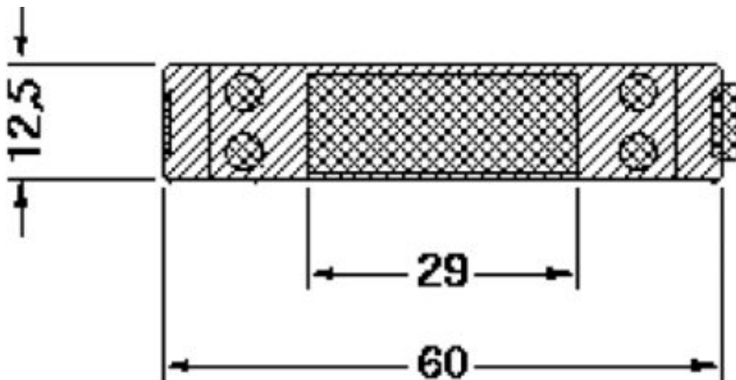
Maßzeichnung
