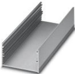
Aufbaugehäuse, Oberteil, Farbe: aluminium, Breite: 130 mm, Bauhöhe: 43,1 mm
