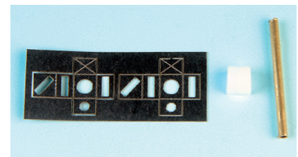
Die Weichenlaterne besteht aus einem weißen Kunststoffblock und der gelaserten Verkleidung. Rechts im Bild sieht man das Führungsröhrchen
