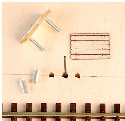
Für den Entkuppelr sind drei Bohrungen unterhalb des Gleises erforderlich. Die Gleismitte ist angezeichnet
