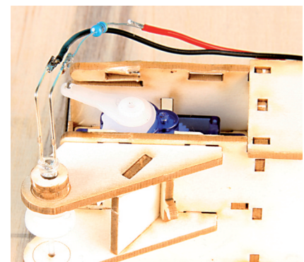
Die LED für die Beleuchtung der Laterne. Der Widerstand und die Litzen müssen selbst angelötet werden
