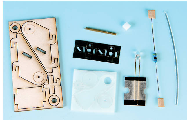
Als Zubehör zum Weichenantrieb wird der Bausatz einer beleuchteten und sich mit der Weichenstellung drehenden Weichenlaterne offeriert
