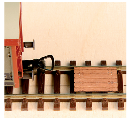
Um den Entkuppelr optimal justieren zu können, sollten Tests mit einigen Fahrzeugen durchgeführt werden
