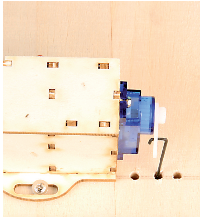
... seitlich aufgesteckt. Das in der Anleitung vorgegebene 8-mm-Longloch war nicht nötig
