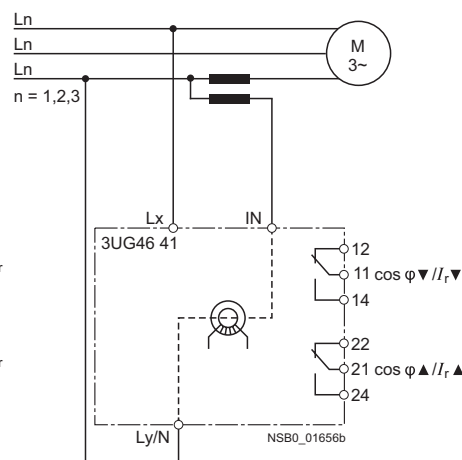
3-phasige Motoren mit Wandler für Ströme > 10 A
