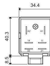
065.07 mit Relais 65.31.x.xxx.xx09
