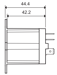
065.05 mit Relais 65.31.x.xxx.xx09
