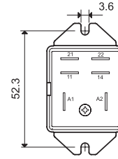
065.05 mit Relais 65.31.x.xxx.xx09
