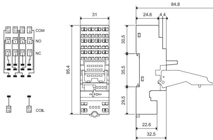
Fassung + Kammbrücke
