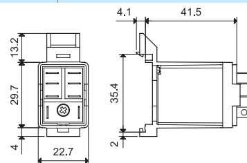
056.27 mit Relais
