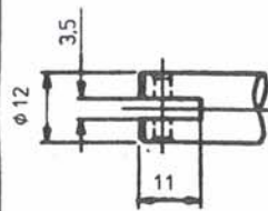
Ankerdetail
