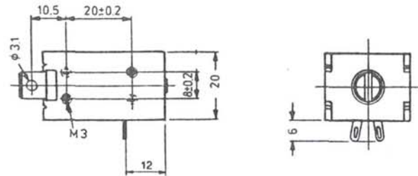
Ankerdetail
