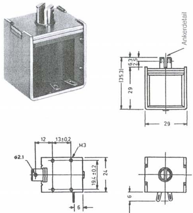
Ankerdetail
