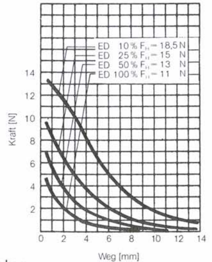
Kraft-Weg-Diagramm F_H = \text{Haltekraft}
