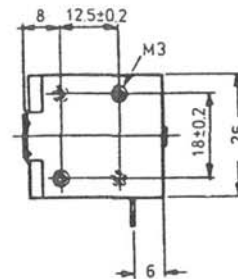
Ankerdetail
