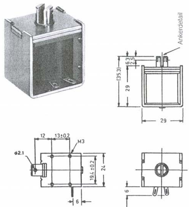
Ankerdetail
