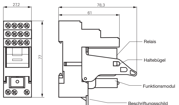
Abmessungen
