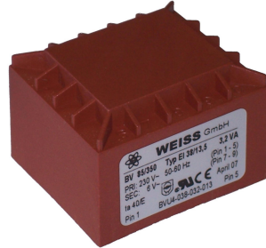
Typ: EI 38 3,2 VA (L x B x H) 41 x 35 x 29 mm
