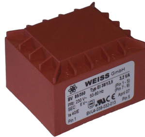
Typ: EI 38/13,5 3,2 VA
