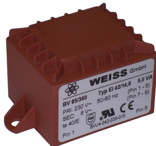
Typ: EI 42/14,8 5,0 VA
