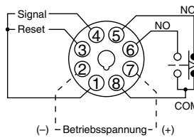
Relais Ausgang
