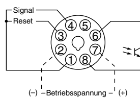
Transistor Ausgang
