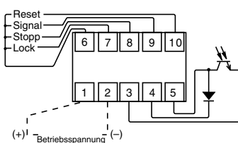
Transistor Ausgang
