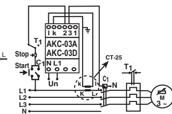
Typ PK 28
