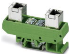
Adapter für PSR-RSM, Hardware- Interface für HTL Encoder - Signalanpassung
