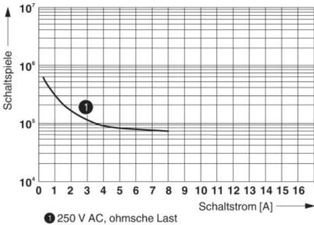
Elektrische Lebensdauer
