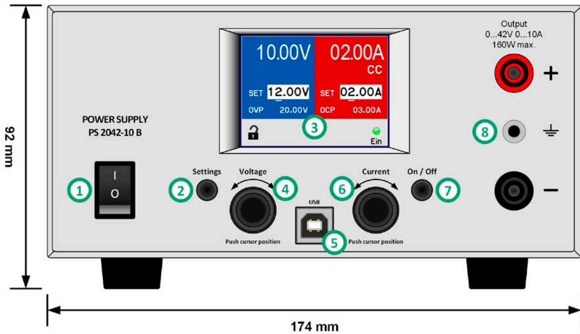
Bild 1 - Vorderseite
