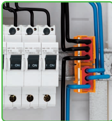
Anschluss ein- und mehrdrähtiger Leiter 6 mm 2
