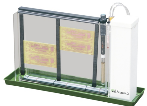
Ätzgerät 2
