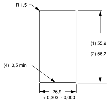
Gehäuseausschnitt ohne Abschirmung
