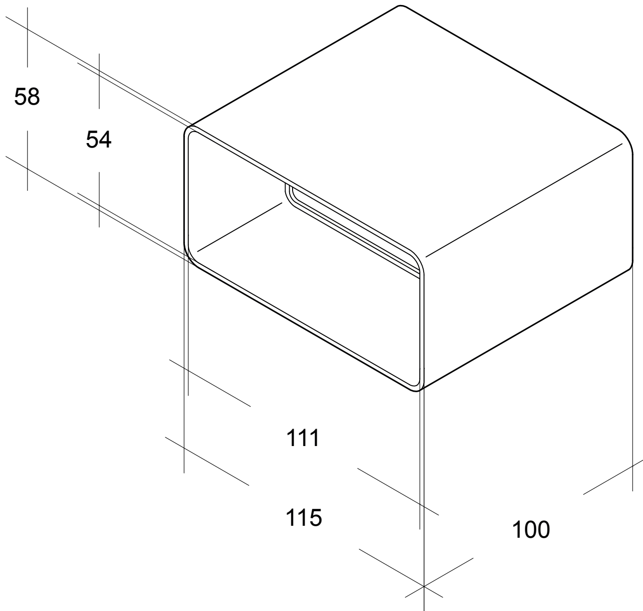
Vierkantrohr-Verbinder 111x54 Material: Kunststoff
