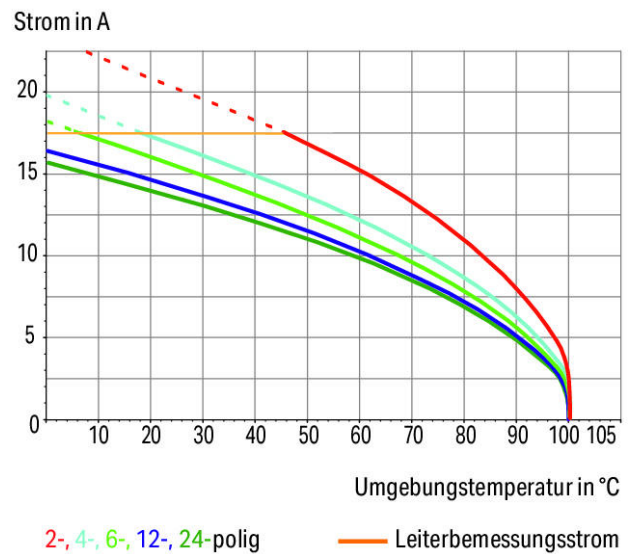
Derating-Kurve 1-Leiter-Federleiste (734-102) mit 1-Leiter-Stiftleiste (734-302) Rastermaß 3,5 mm / Leiterquerschnitt 1,5 mm 2 „f“ In Anlehnung an: EN 60512-5-2 / Reduktionsfaktor 0,8
