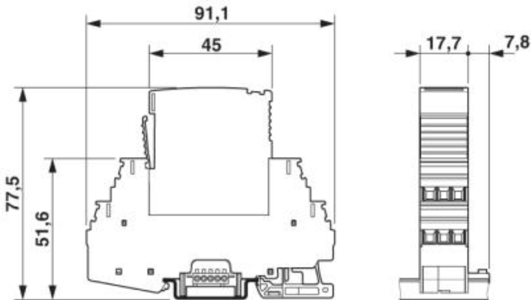
Maßzeichnung
