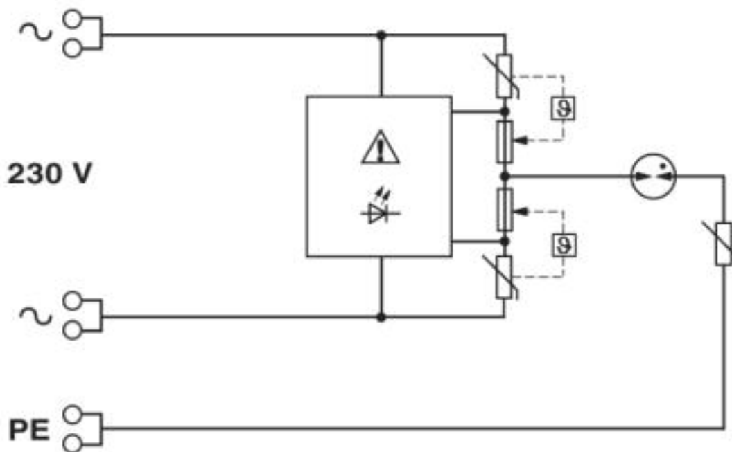
Schaltplan
