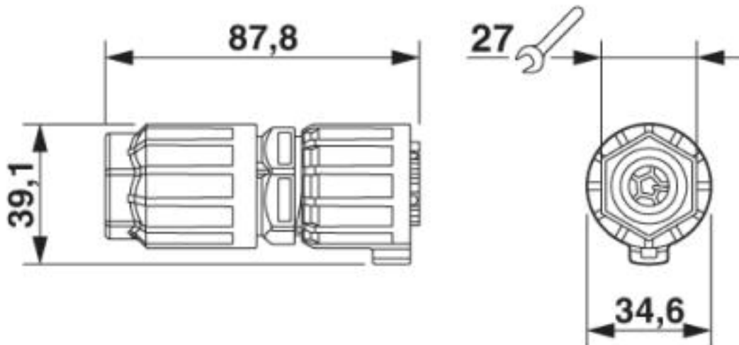
Maßzeichnung
